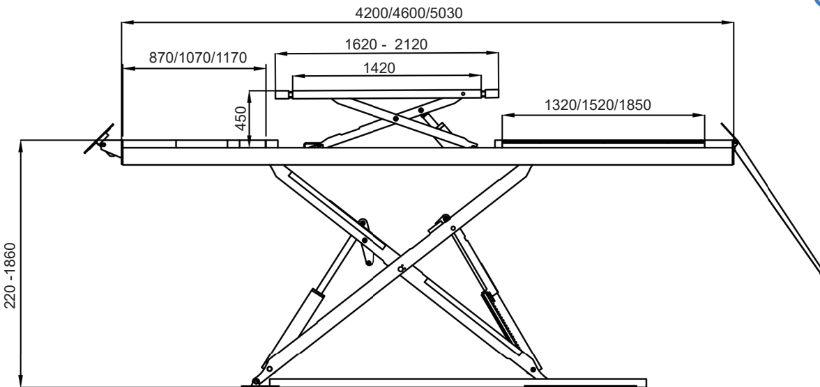
ROLLING JACK 2T / 3 T ROLLING JACK 2T / 3T OPTIONAL
